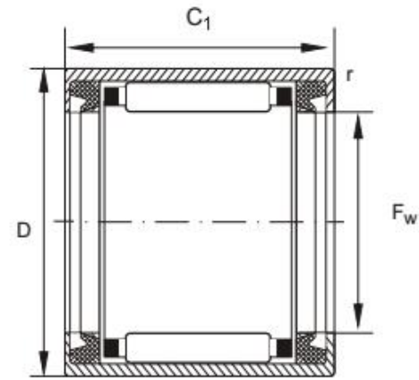
HK..2RS
